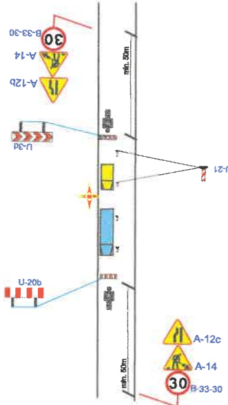
schemat dla prac postępujących dla wymiany słupów oświetlenia drogowego
